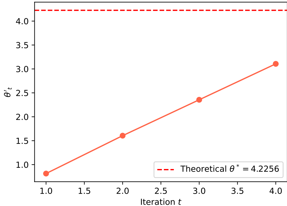
CE Method: Parameter sequence \theta'_t
