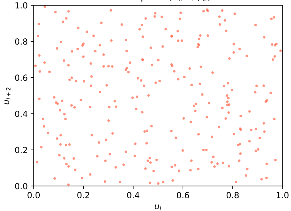
PCG64 pairs (u_i, u_{i+2})
