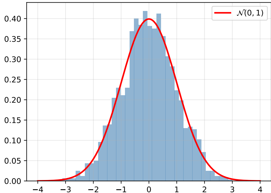
Box-Muller: Z_2
