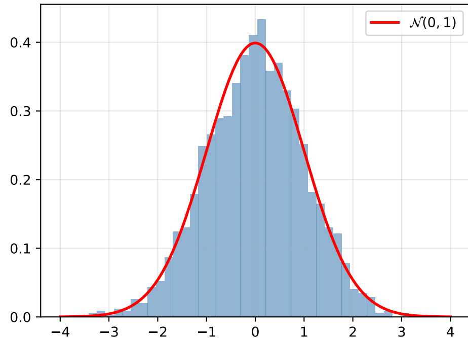
Box-Muller: Z_1
