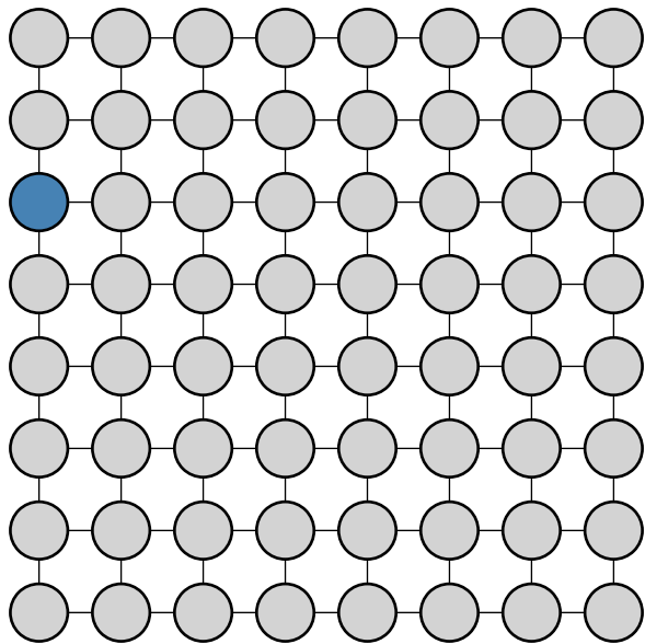
Step 2 (1 particles)
