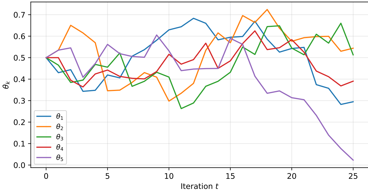
CE knapsack: parameter evolution \theta_k (first 5 coords)
