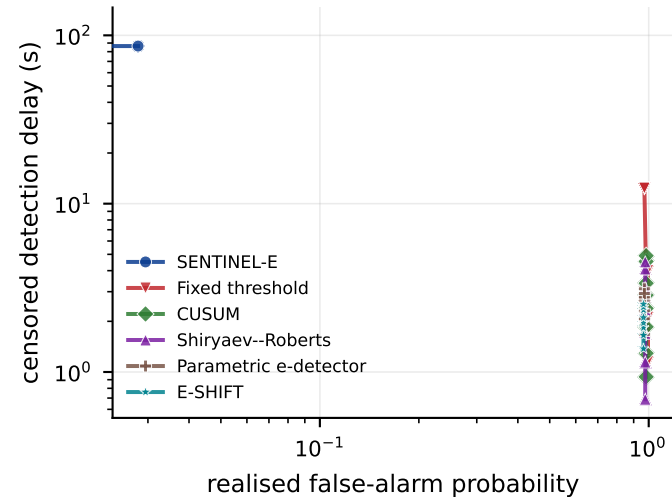
(a) UCSD Ped2 (lag=5)
