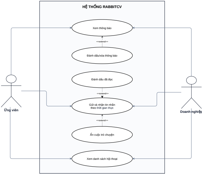
Hình 4.4: Đặc tả usecase giao tiếp và thông báo
