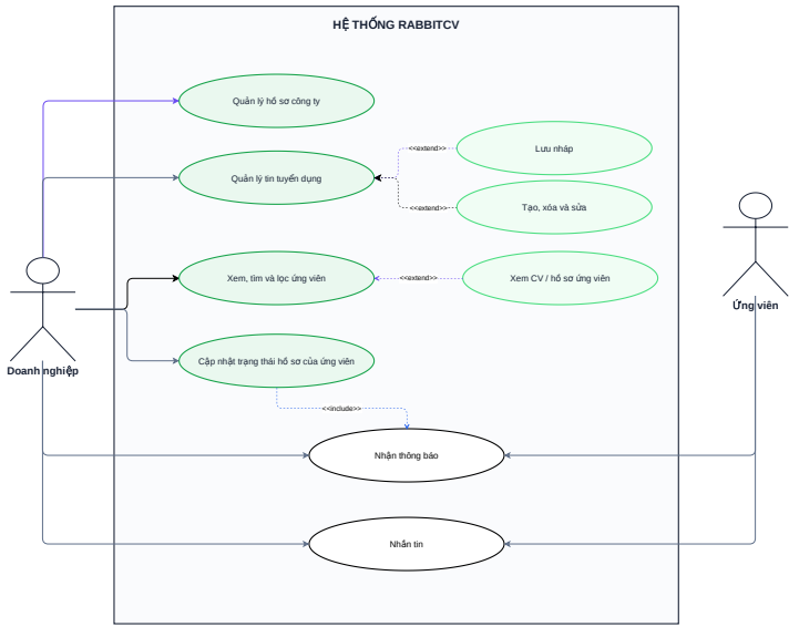
Hình 4.5: Đặc tả usecase quản lý thông tin doanh nghiệp
