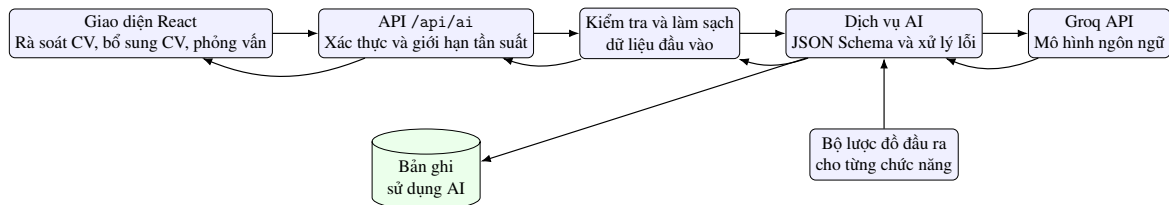
Hình 6.1: Kiến trúc tổng quát của mô-đun AI
