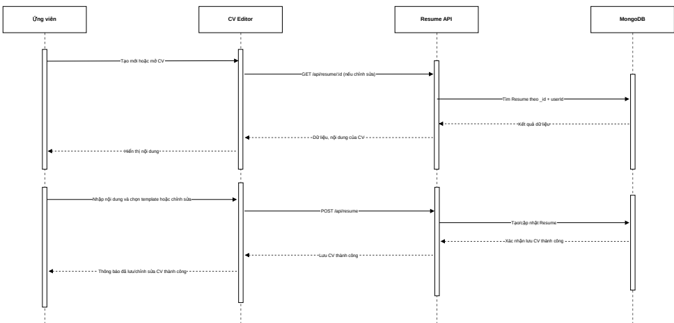
Hình 4.15: Lược đồ tuần tự: Quản lý CV
