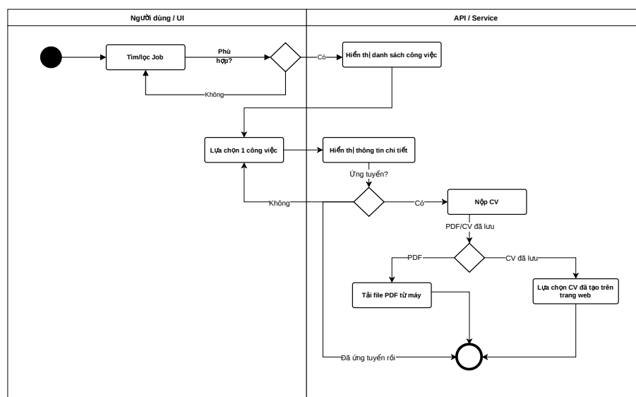
Hình 4.9: Lược đồ hoạt động: Tìm kiếm việc làm
