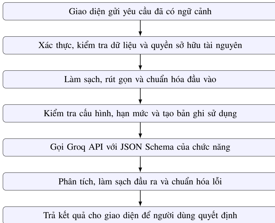
Hình 6.2: Quy trình xử lý một yêu cầu AI
