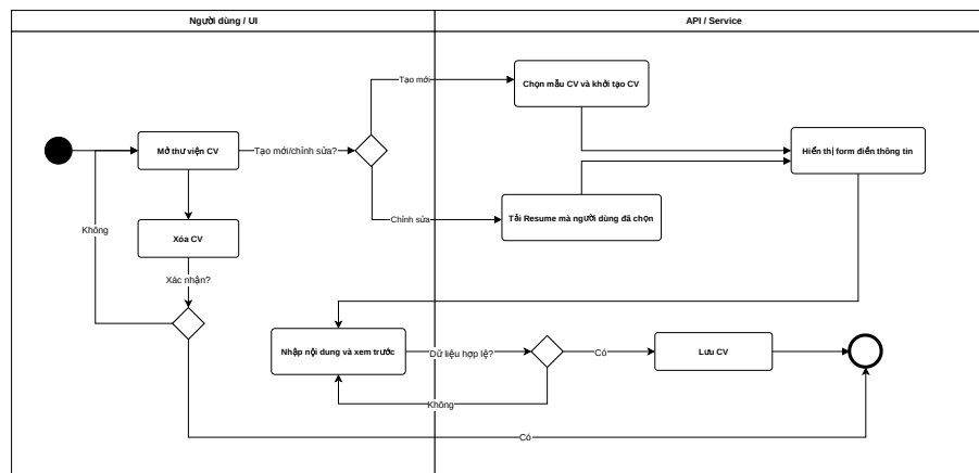
Hình 4.8: Lược đồ hoạt động: Quản lý CV
