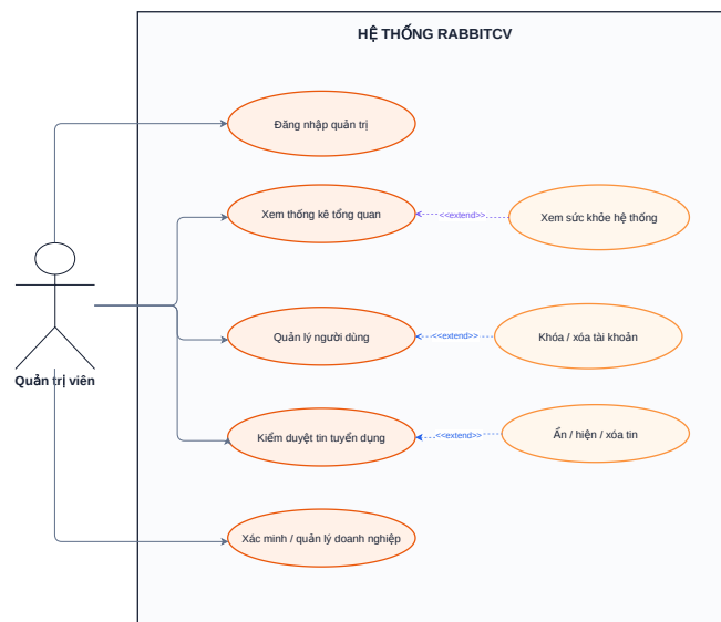
Hình 4.6: Đặc tả usecase phân hệ Quản trị viên
