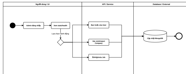
Hình 4.13: Lược đồ hoạt động: Quản trị viên
