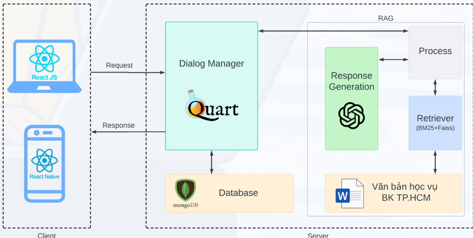
Hình: Kiến trúc chatbot
