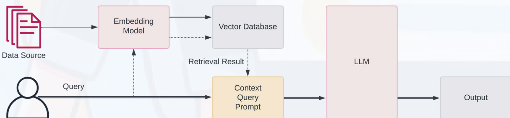
Hình: Kỹ thuật RAG
