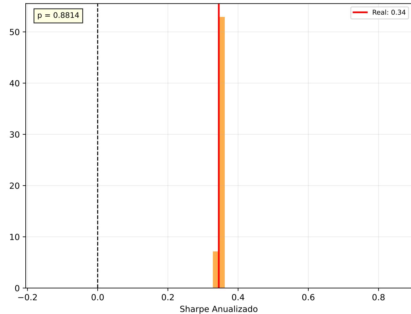
c) Monte Carlo — ITUB4.SA
