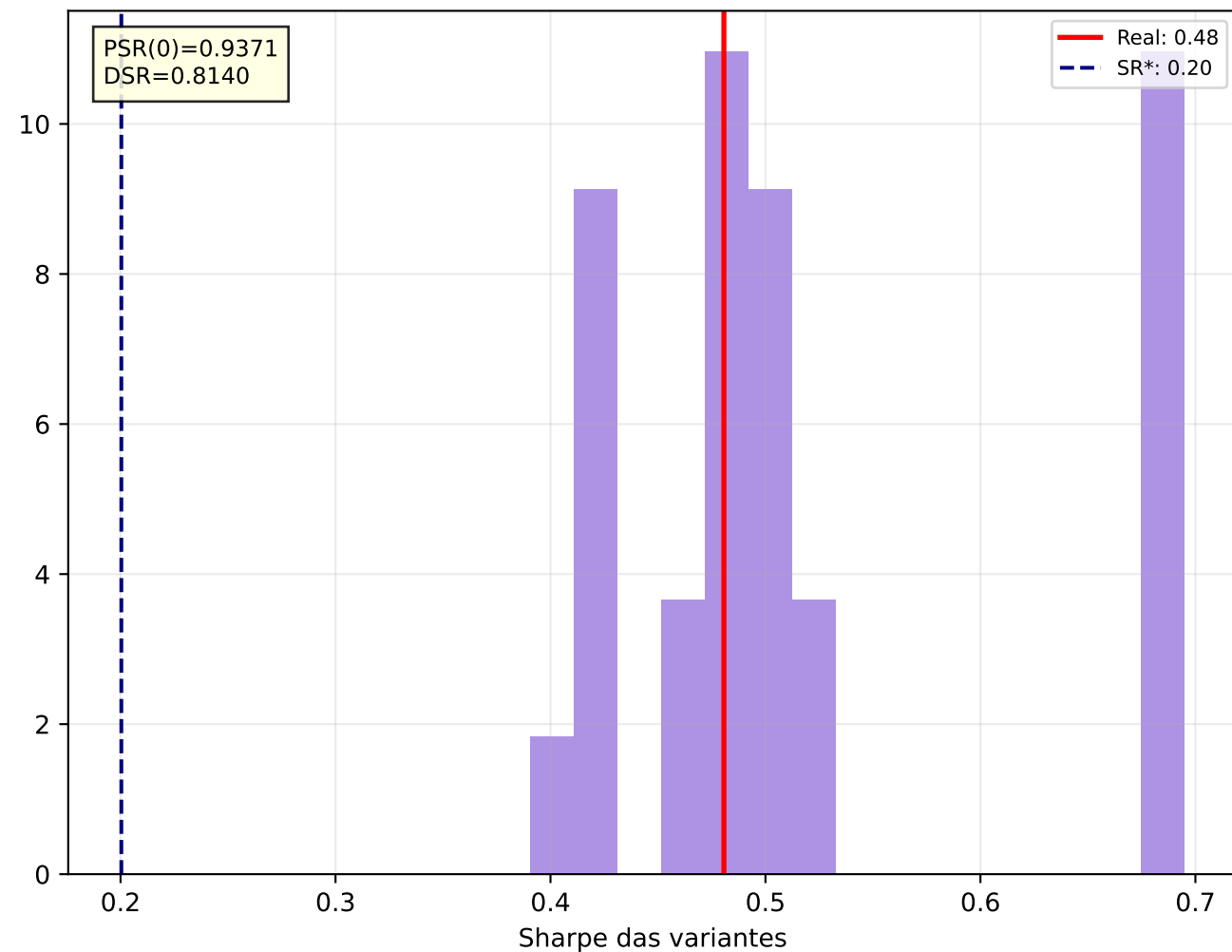
d) DSR — WEGE3.SA
