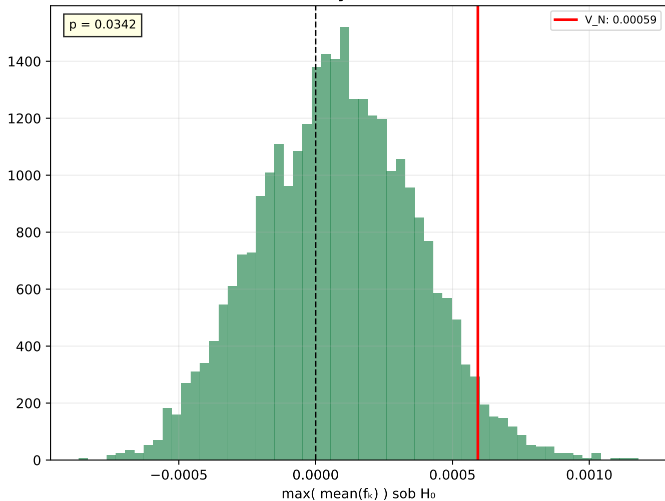
e) White's Reality Check — WEGE3.SA
