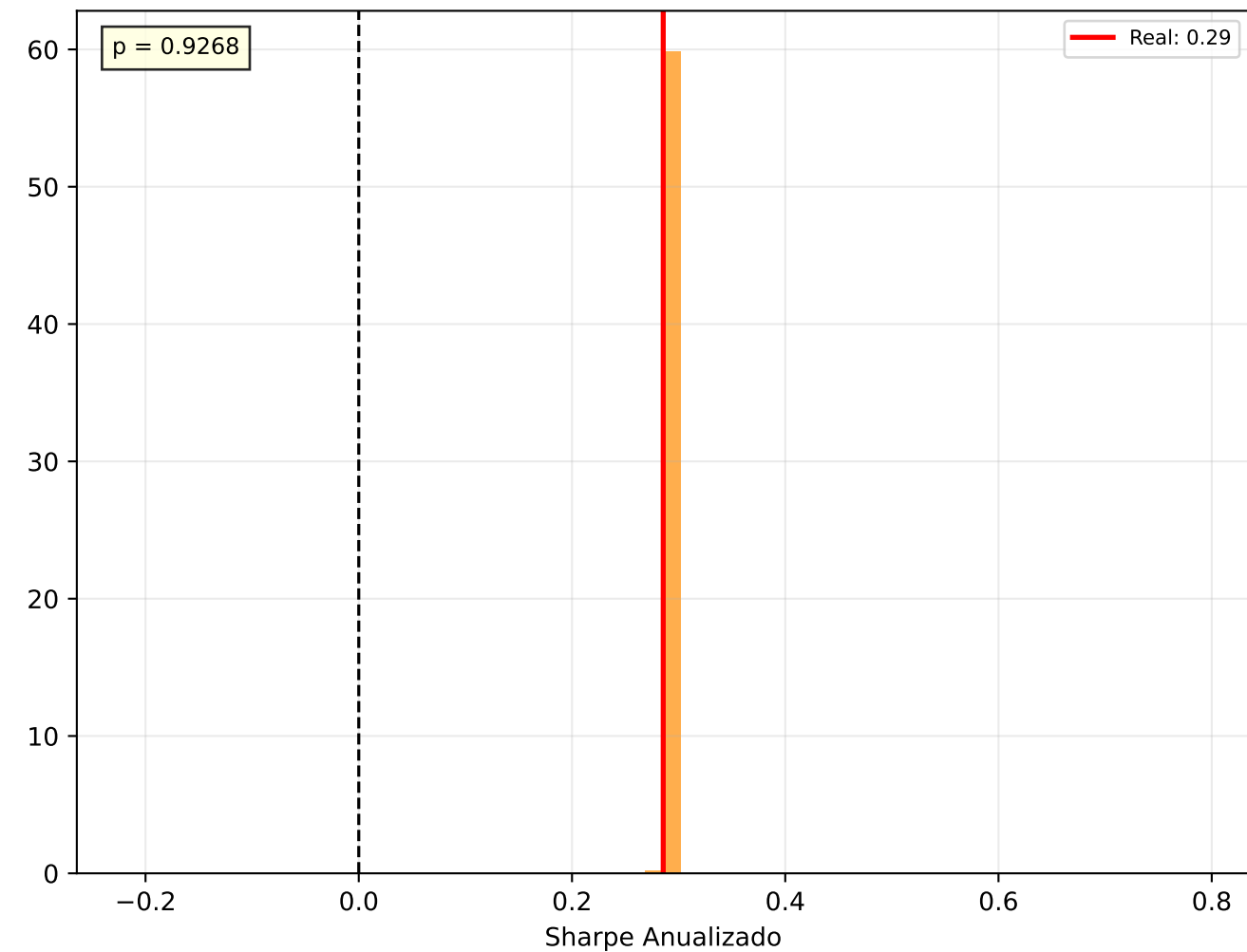
c) Monte Carlo — VALE3.SA
