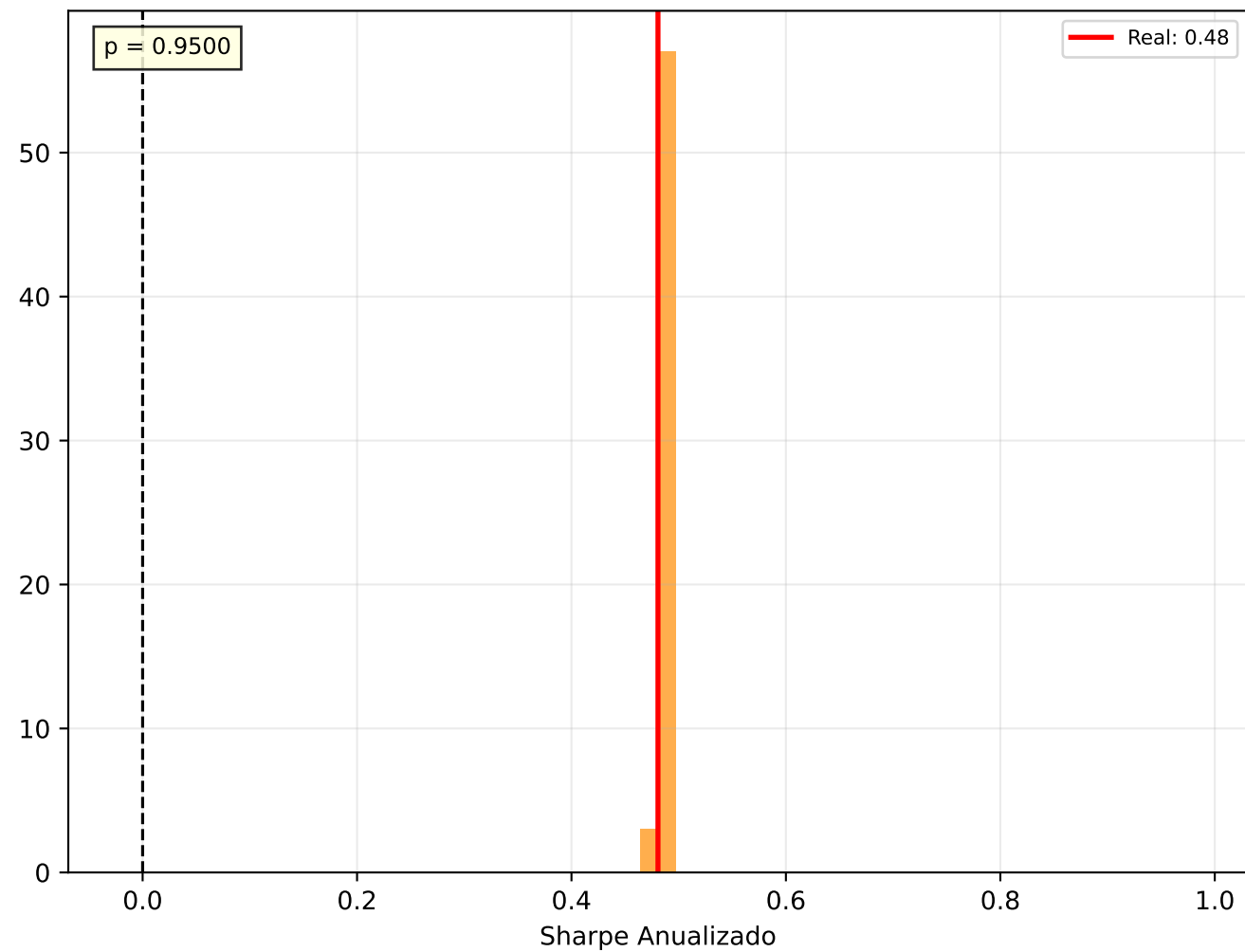
c) Monte Carlo — WEGE3.SA
