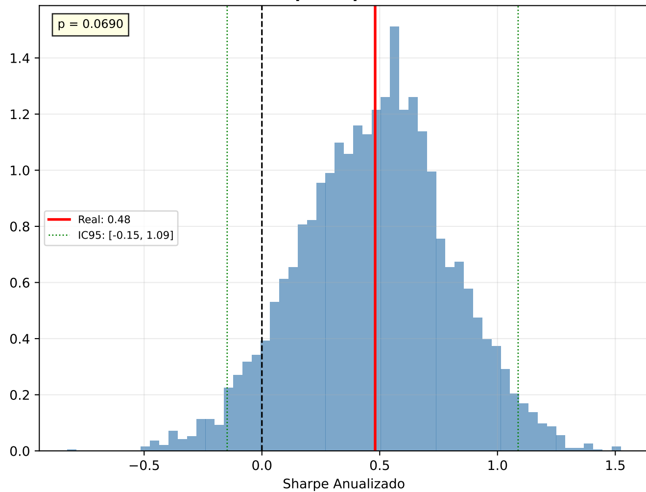
b) Bootstrap Sharpe — WEGE3.SA
