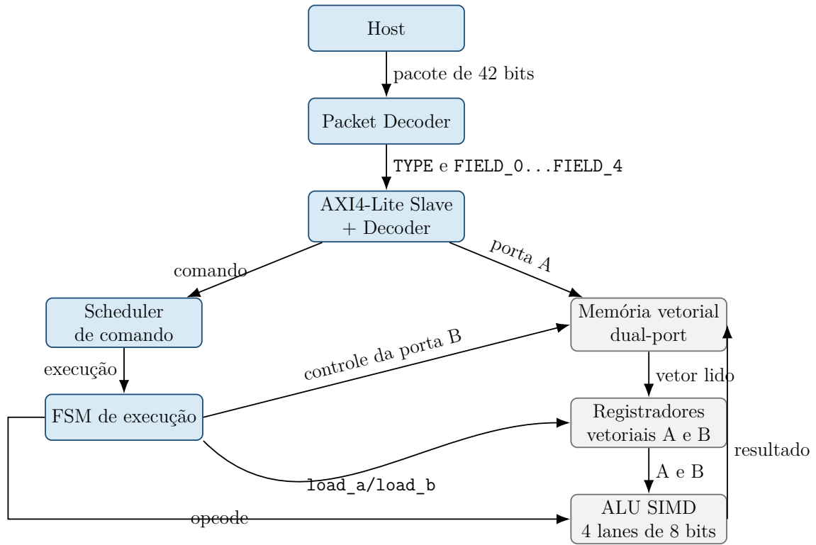
Figure 1: Arquitetura funcional da mini GPU SIMD.
