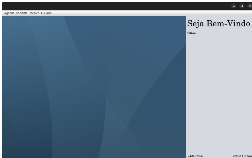
Figura 3: Tela Inicial
