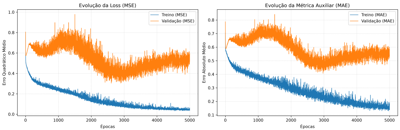
Figure 5: Convergência da MLP Baseline com Regularização L1 ( \lambda = 10^{-5} ).
