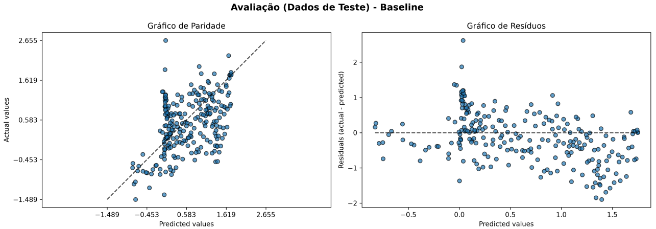
Figure 7: Avaliação no teste (Modelo Baseline): Gráfico de Paridade e Distribuição de Resíduos.
