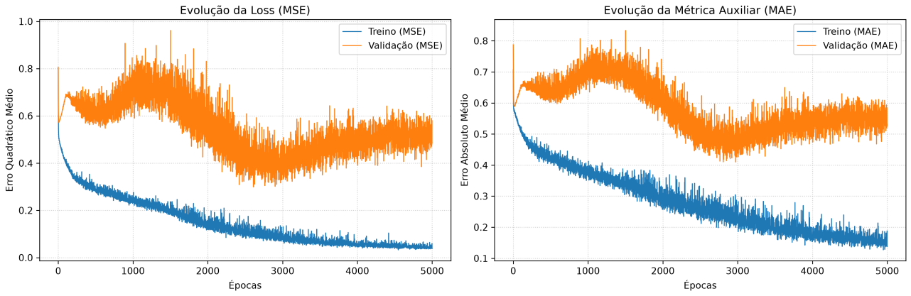
Figure 4: Convergência da MLP Baseline com Regularização L2 ( \lambda = 10^{-6} ).
