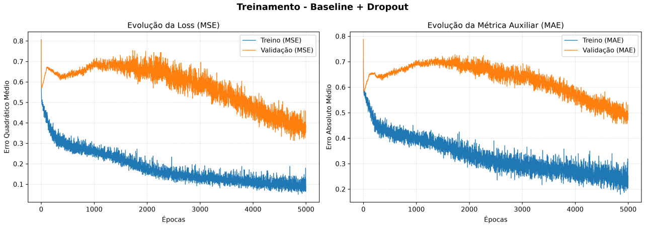
Figure 6: Convergência da MLP Baseline com Dropout ( p_1 = 0.1, p_2 = 0.05 ).
