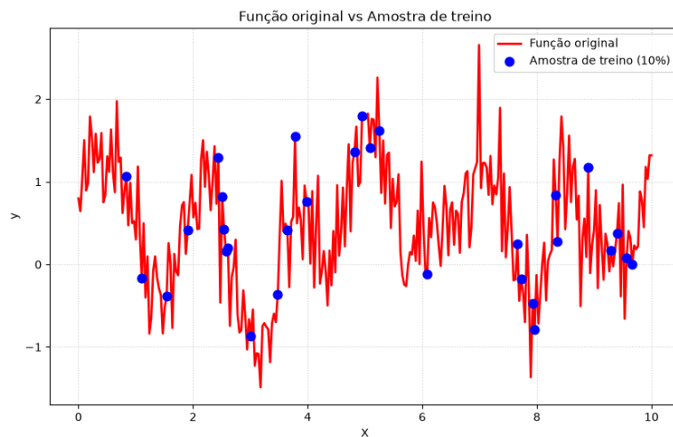
Figure 1: Função original vs Amostra de treino
