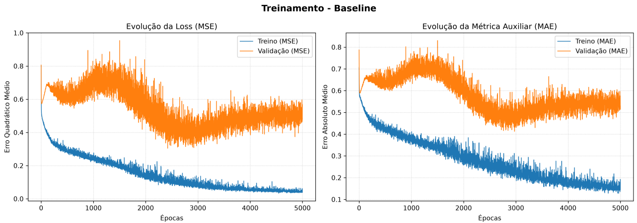
Figure 2: Convergência da MLP Baseline (Vanilla).
