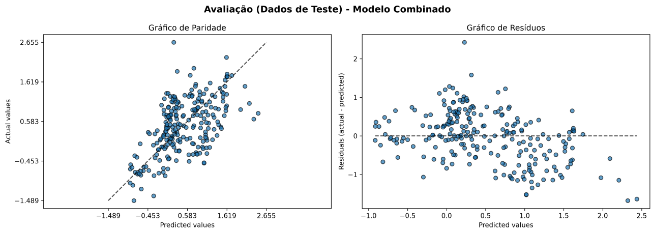
Figure 8: Avaliação no teste (Modelo Combinado): Gráfico de Paridade e Distribuição de Resíduos.
