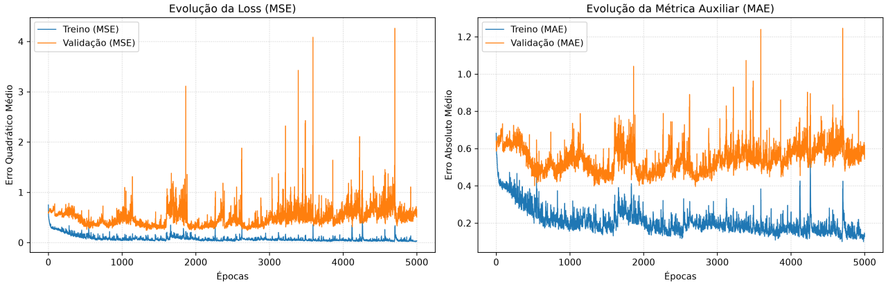
Figure 3: Convergência da MLP Baseline com Momentum ( \beta = 0.9 ).
