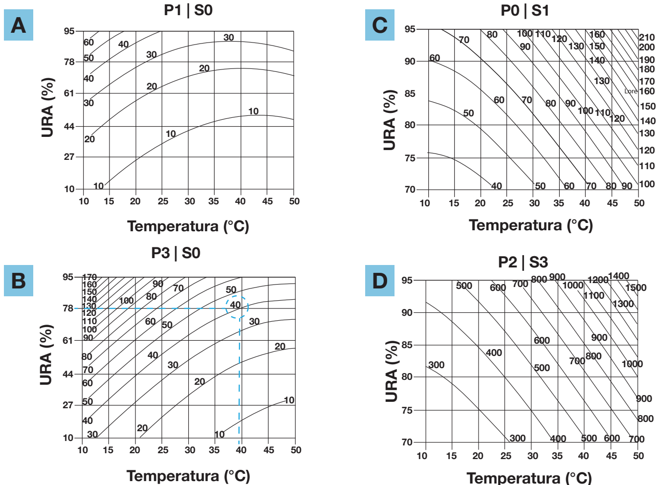
Figura 1: Efeito das características ambientais e climáticas sobre o aço-carbono.
