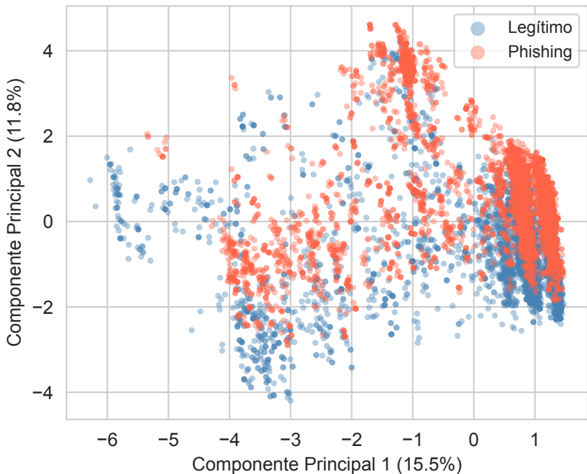
PCA 2D — Conjunto de Treino
