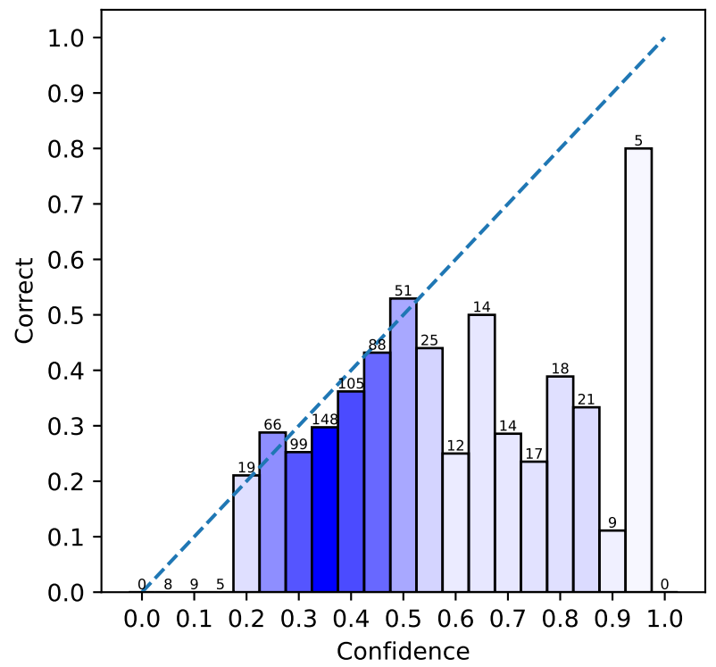
IGLB
