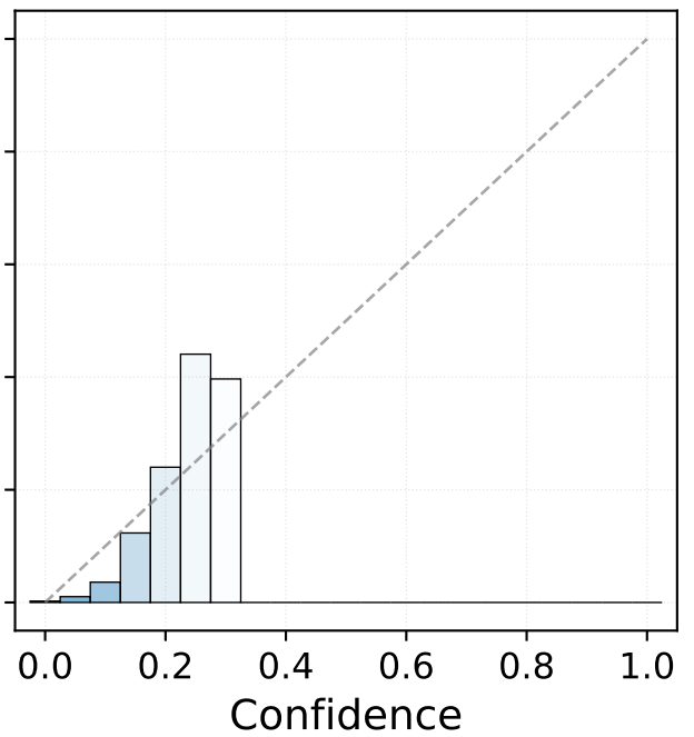
LINR
