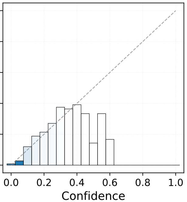
IGLB
