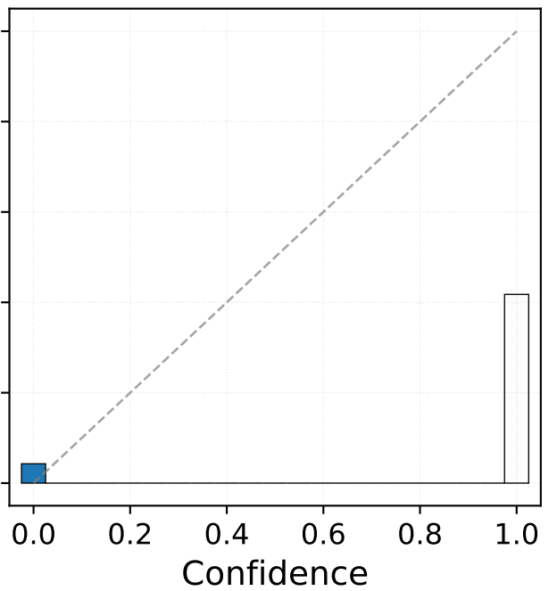
LOGR
