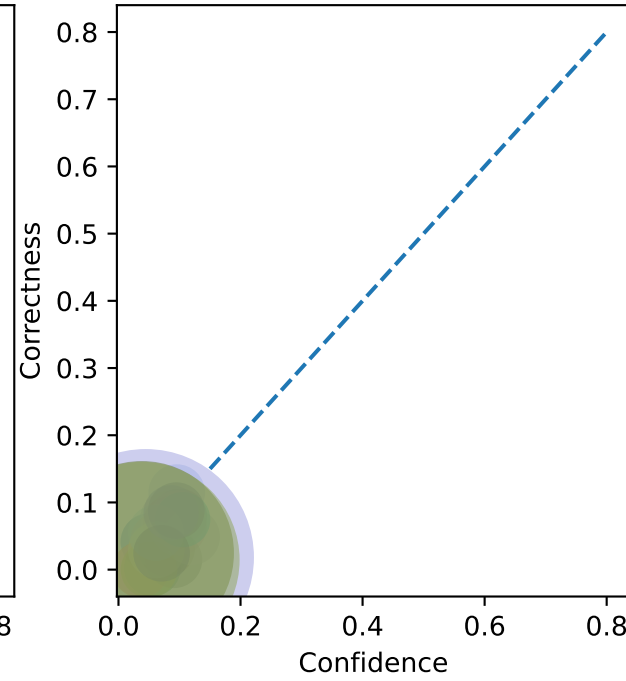
IGLB
