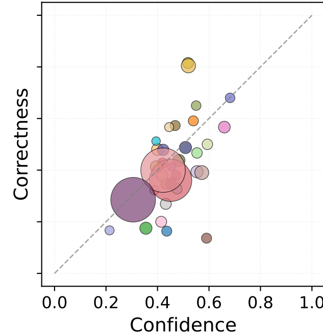
IGLB
