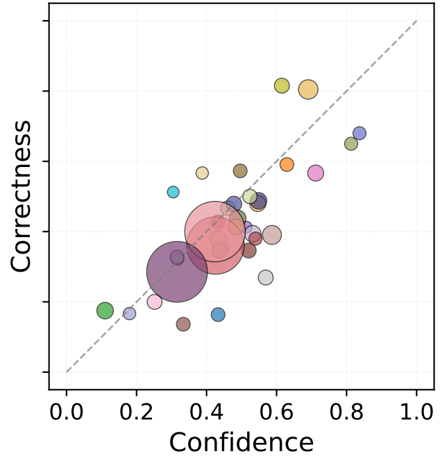
LINR
