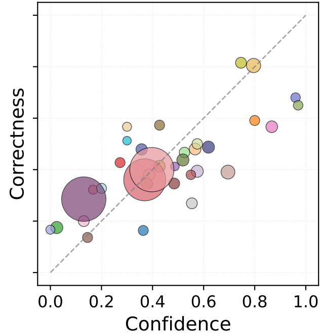
LOGR
