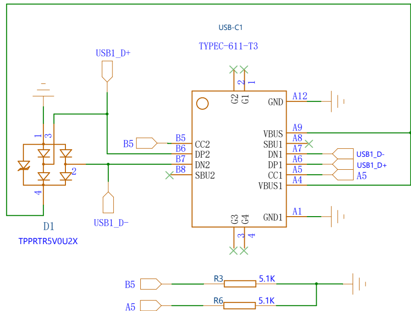
TYPE-C电路
