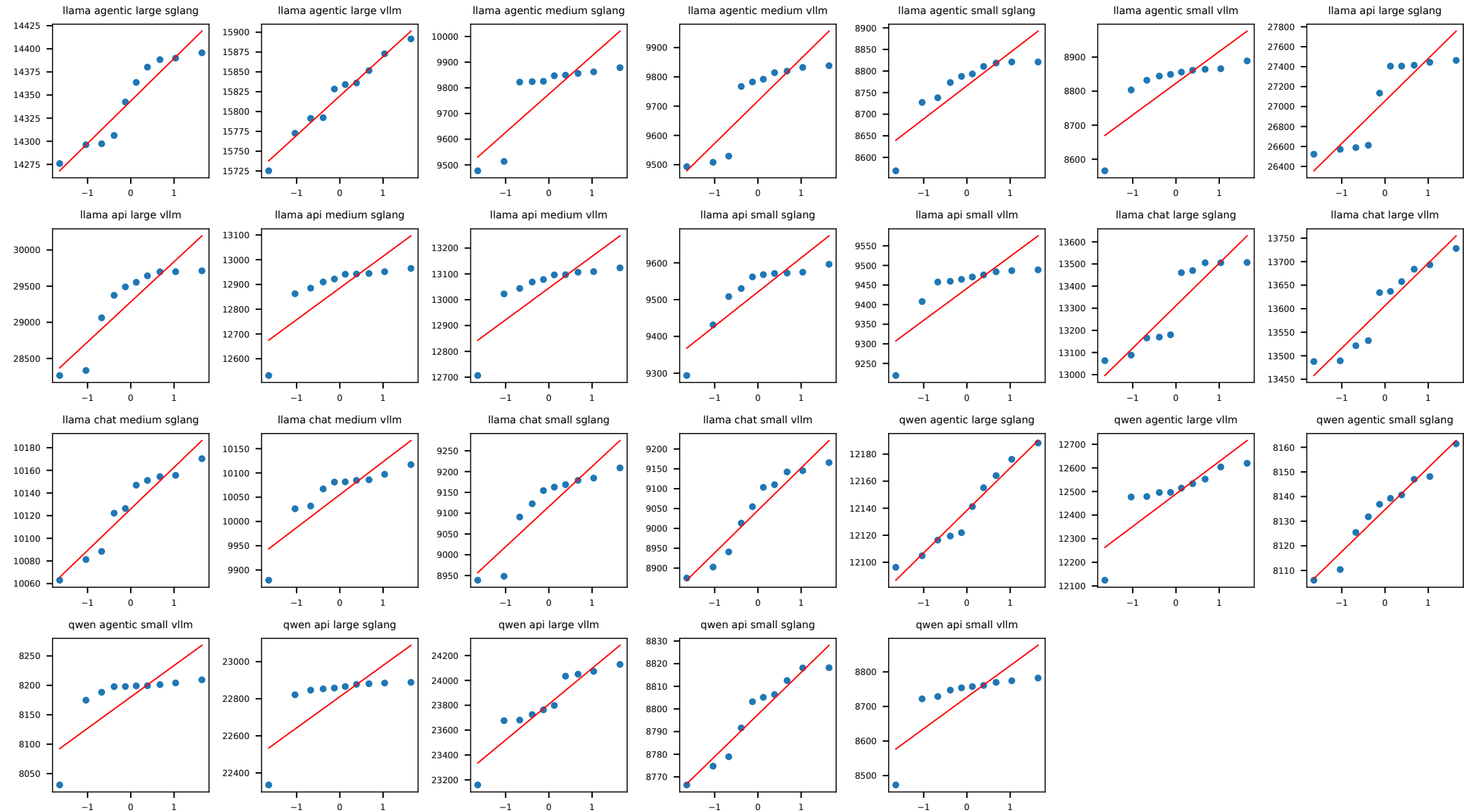
Normal Q-Q plots: e2e_ms_median
