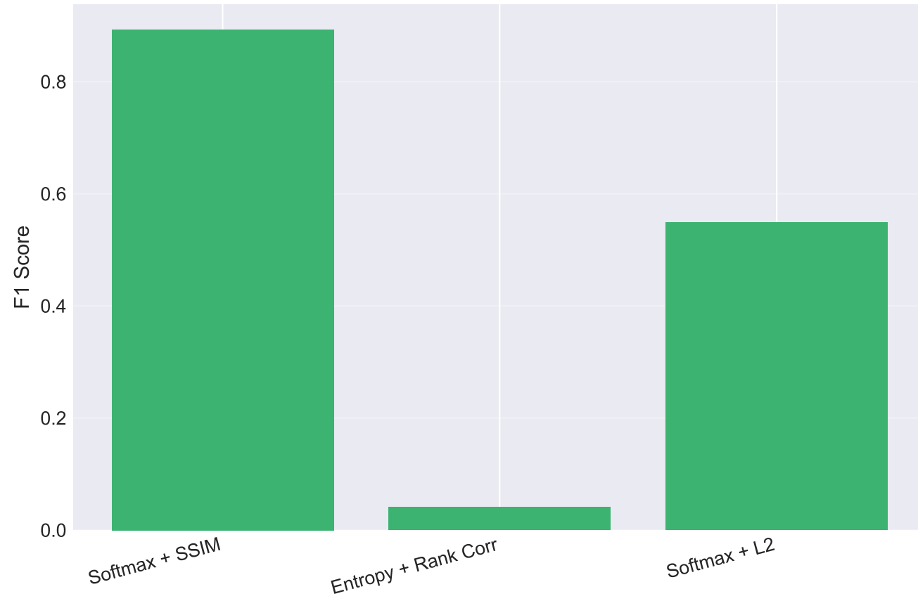
(c) F1 Score
