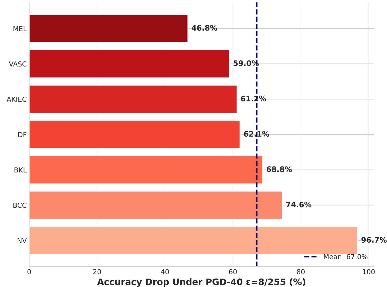
(d) Class-wise Attack Success Rate
