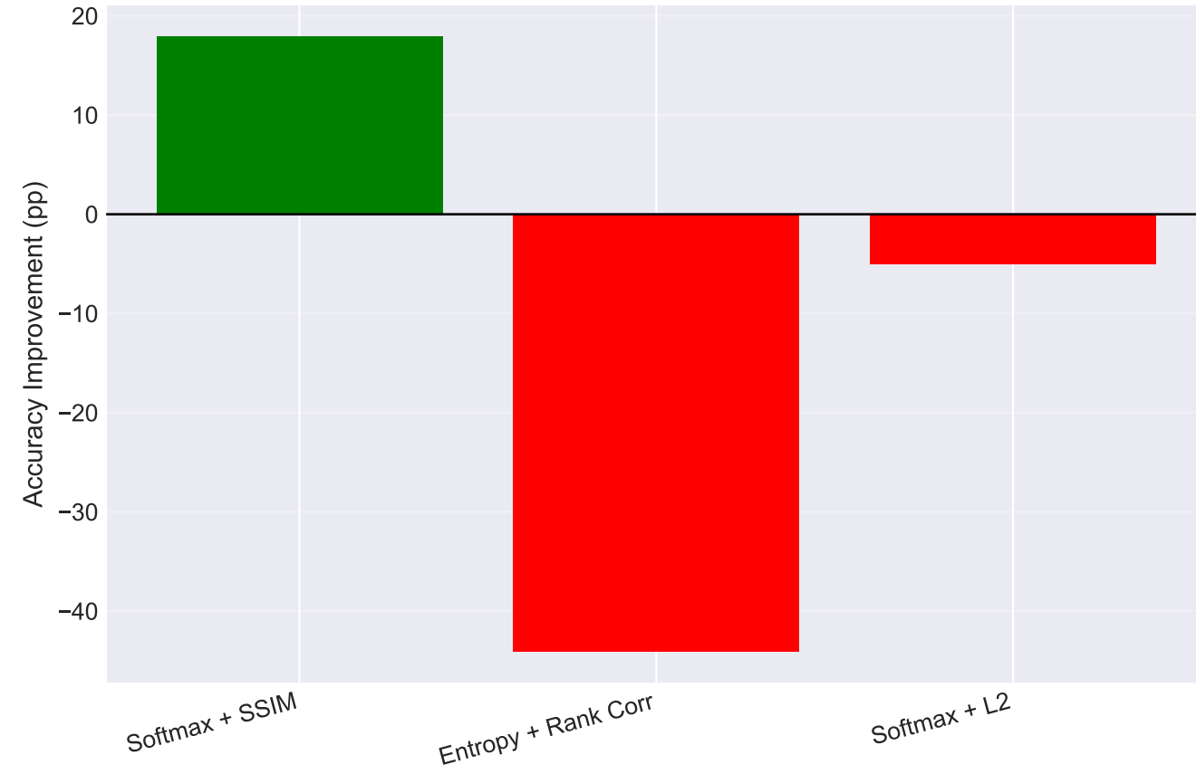
(d) Improvement over Baseline
