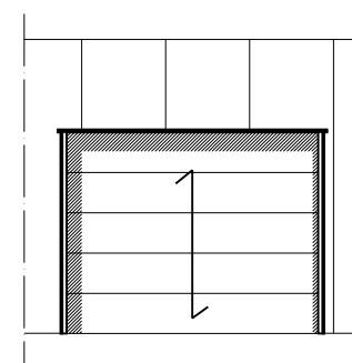
- VOORGEVEL -
