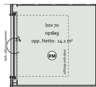
- PLATTEGROND -
