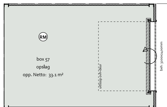
- PLATTEGROND -
