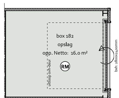
- PLATTEGROND -
