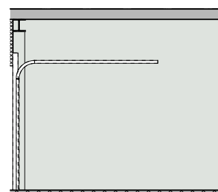
- DOORSNEDE -
