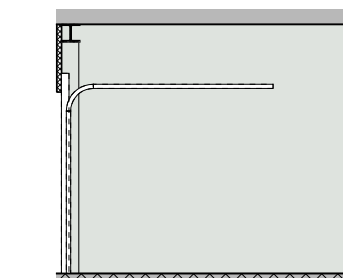
- DOORSNEDE -
