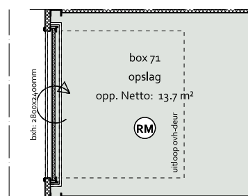
- PLATTEGROND -
