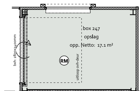
- PLATTEGROND -
