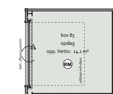
- PLATTEGROND -
