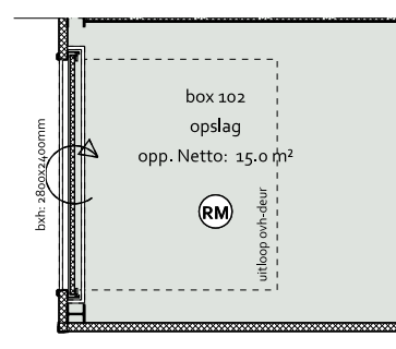
- PLATTEGROND -
