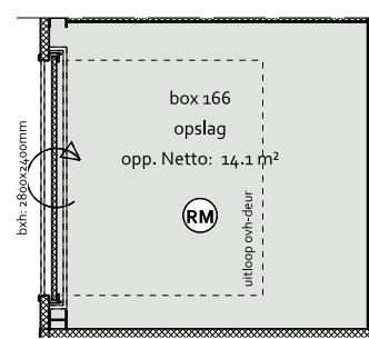
- PLATTEGROND -
