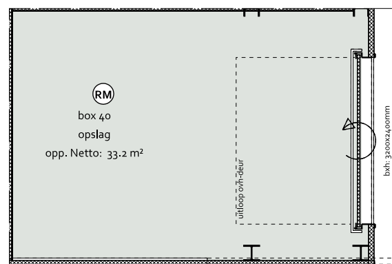
- PLATTEGROND -
