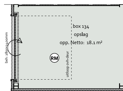
- PLATTEGROND -
