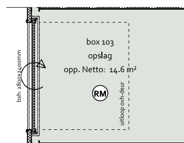
- PLATTEGROND -
