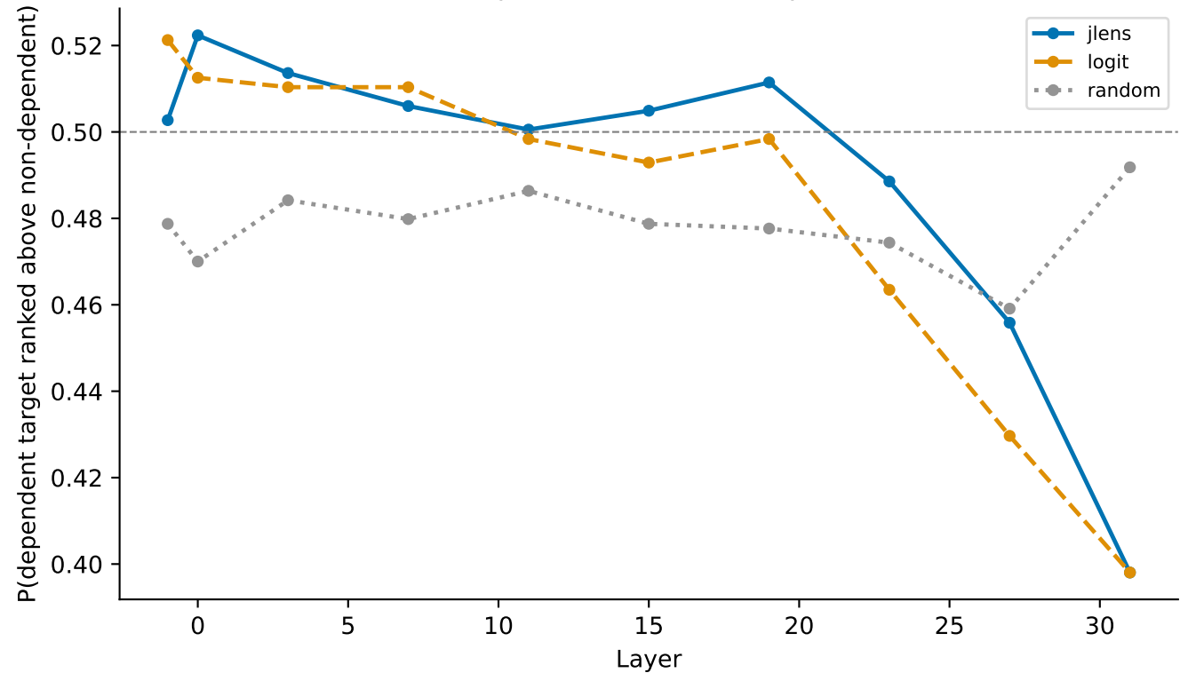
E10-3 control dependence, all — deepseek-coder-6.7b
