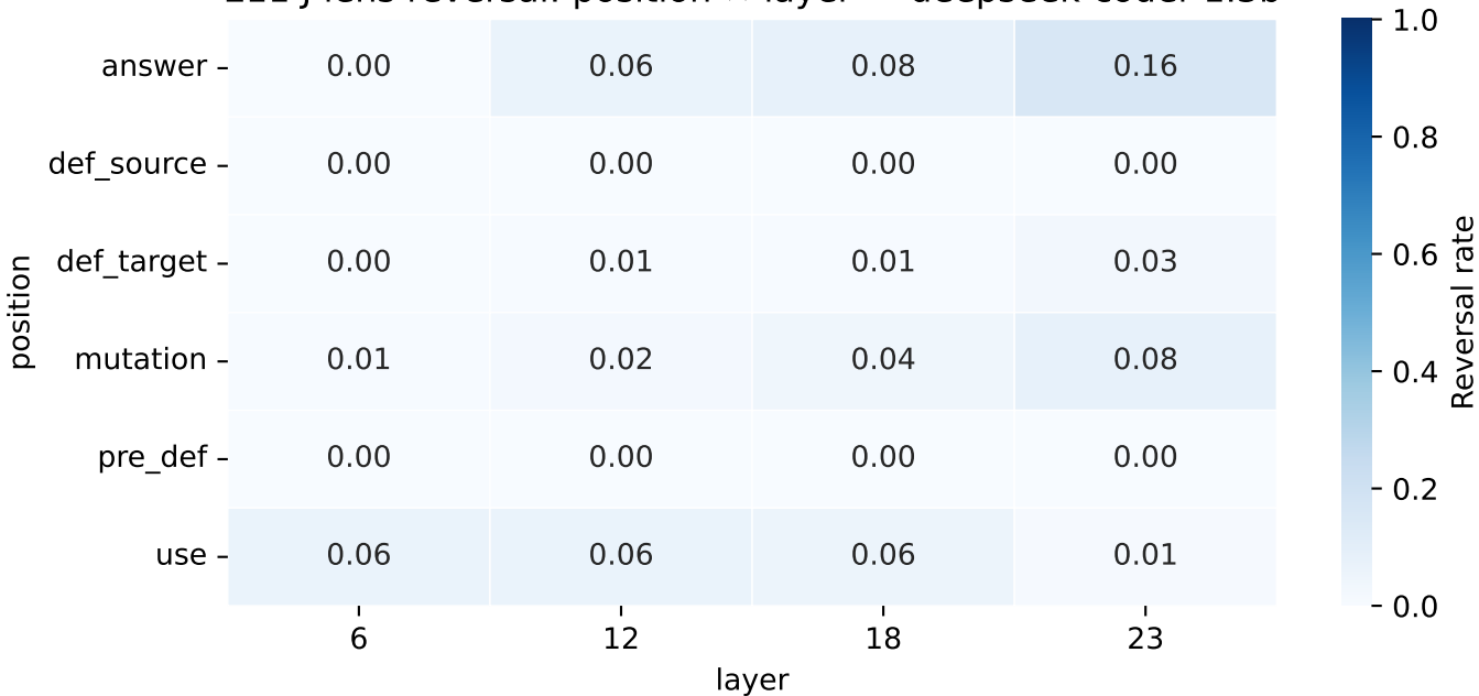
E11 J-lens reversal: position × layer — deepseek-coder-1.3b
