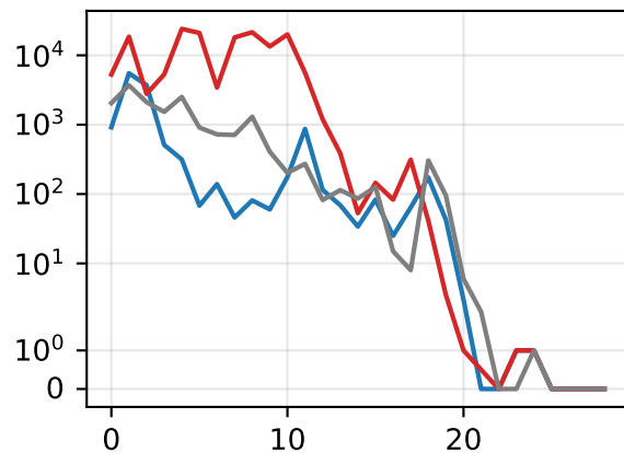
loopvar
