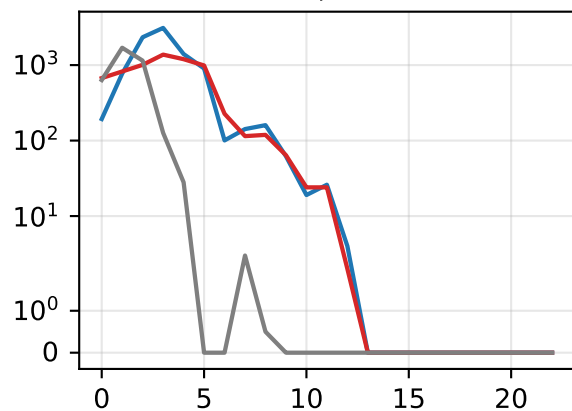
loopvar
