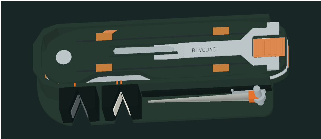
Vue de principe en coupe; certains éléments extérieurs sont masqués.
