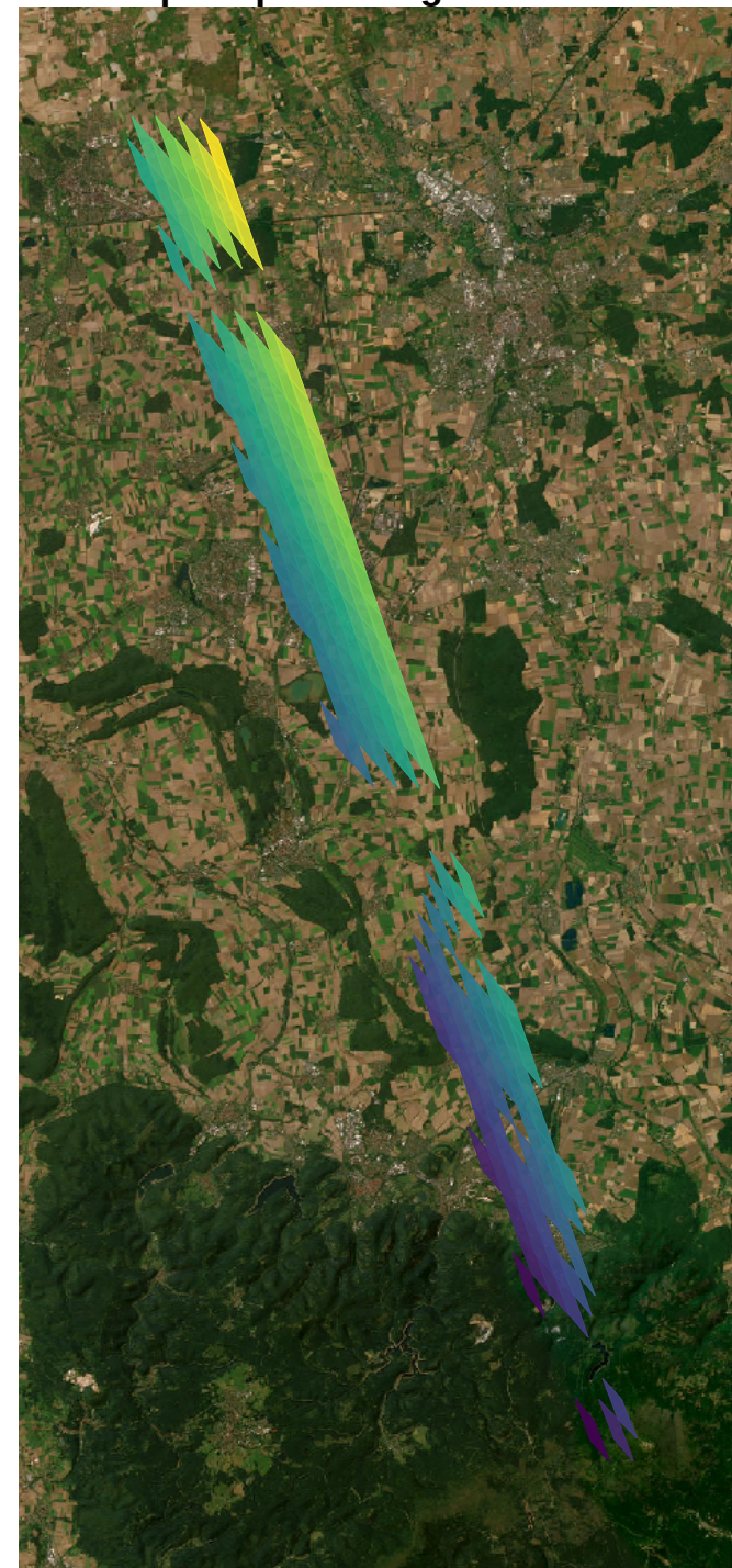
SIF footprint phase angle
