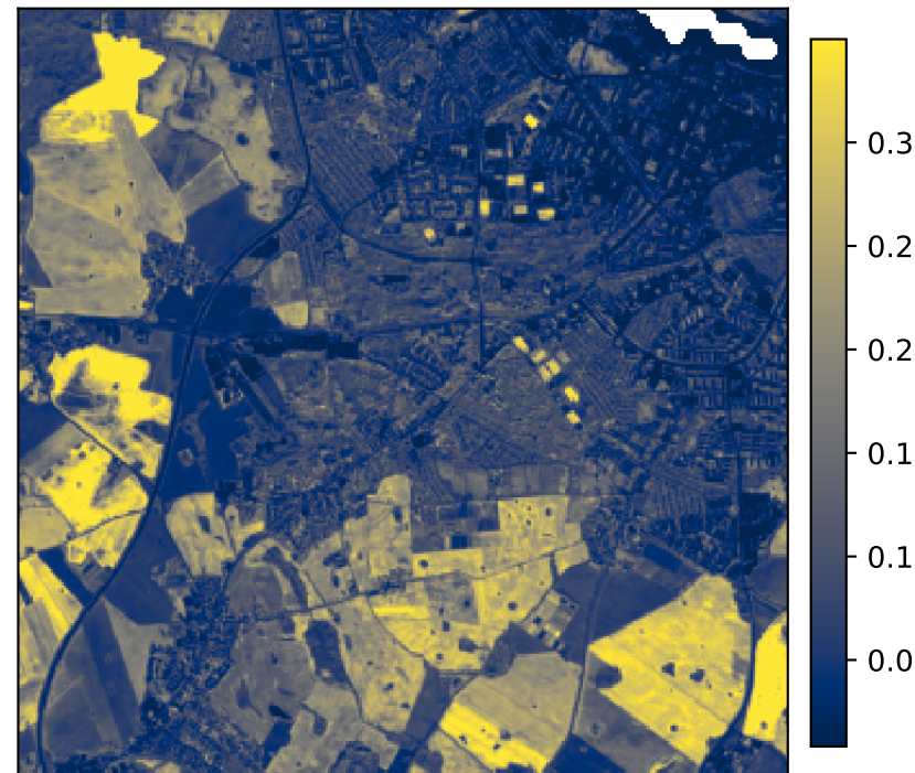
7: apar valid=1.000
