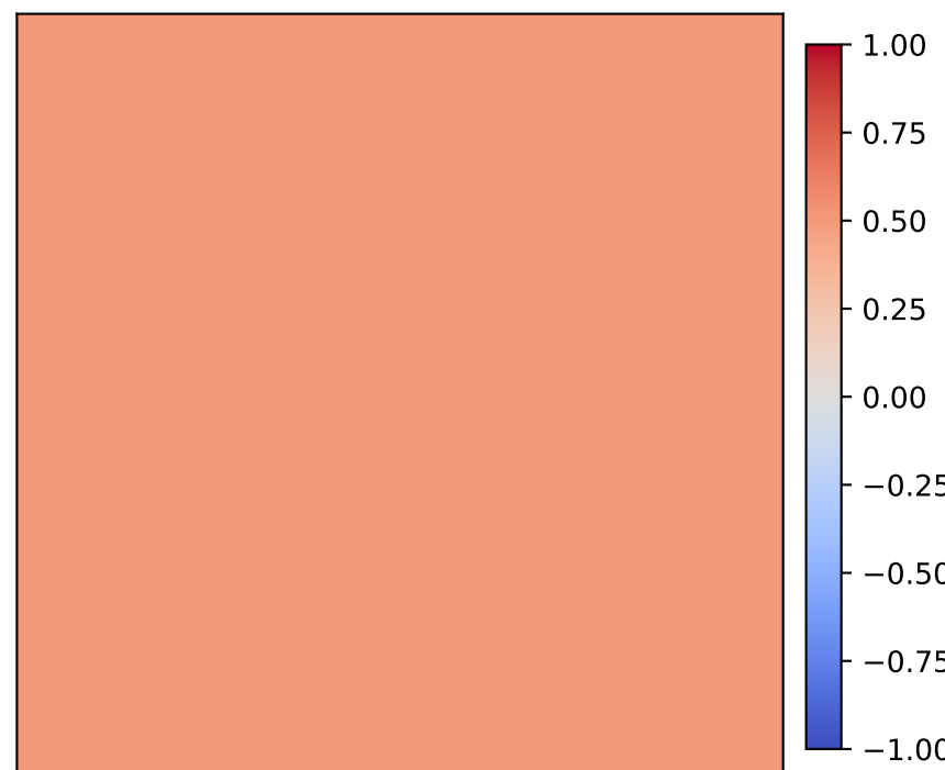
18: month_cos valid=1.000
