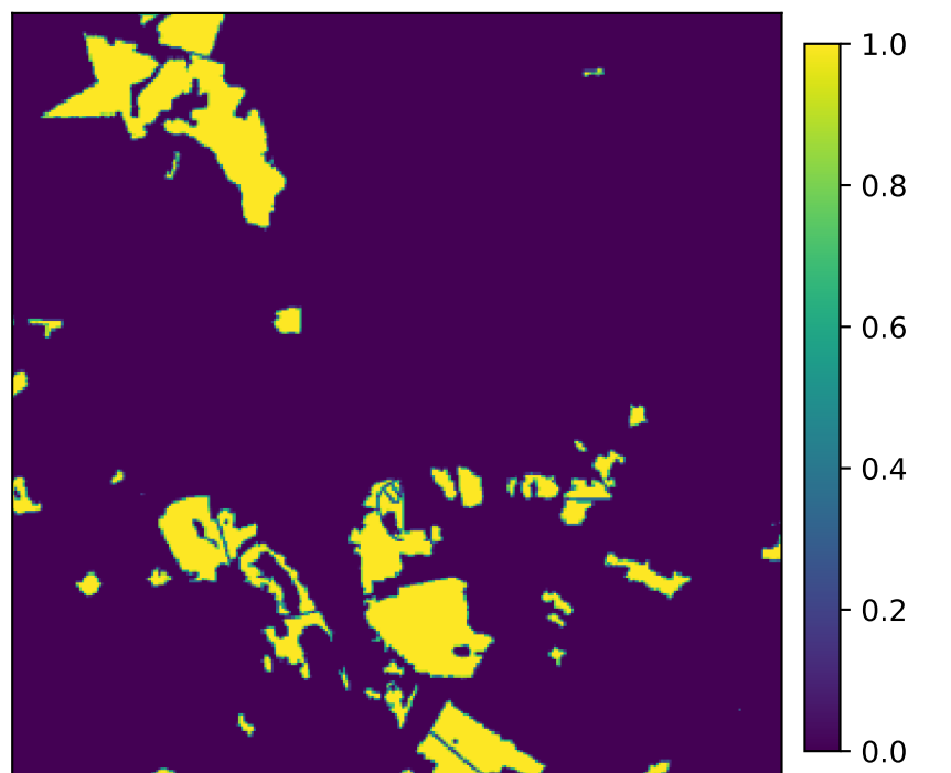
16: non_crop_fraction valid=1.000
