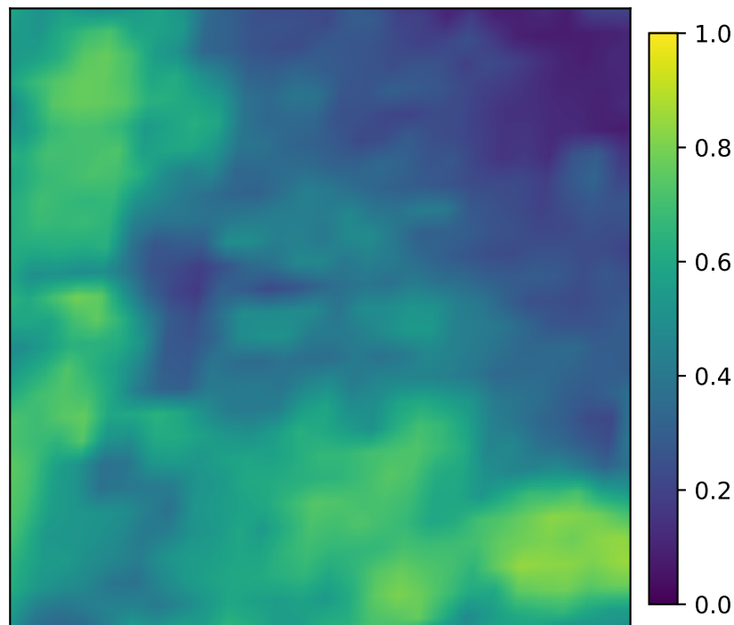
9: winter_barley_fraction valid=1.000
