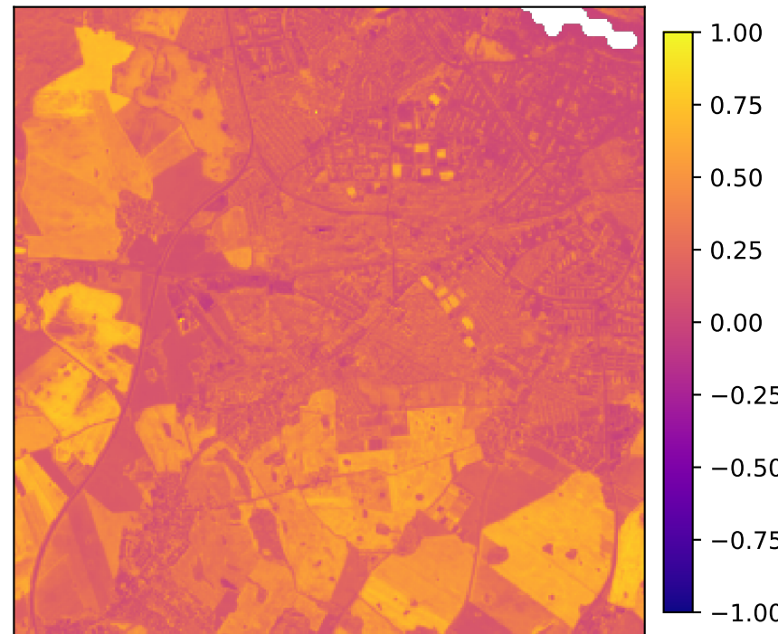
6: par valid=1.000
