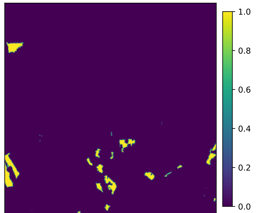
14: other_crop_fraction valid=1.000
