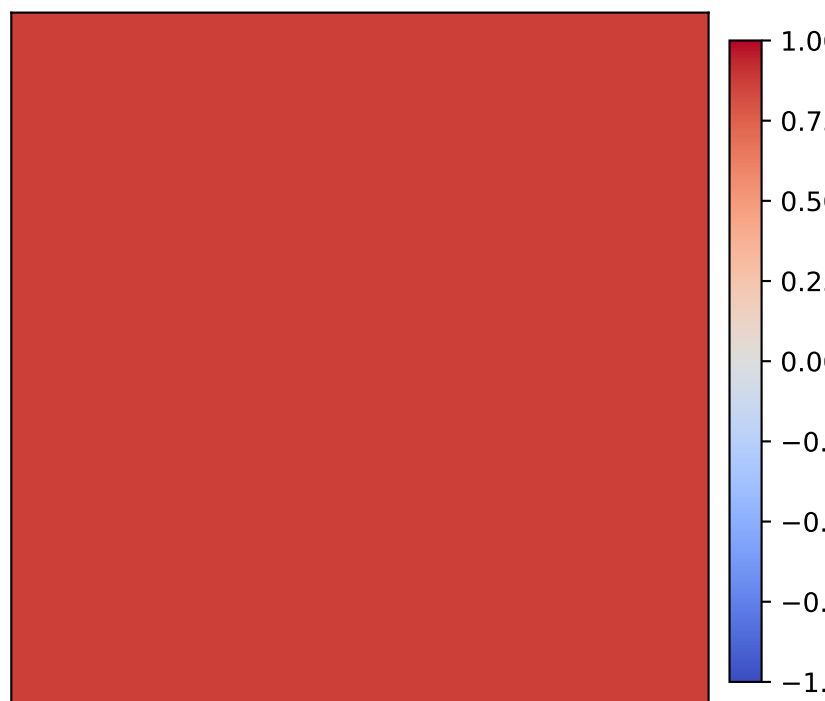
17: month_sin valid=1.000
