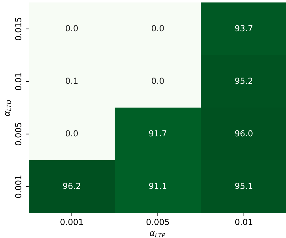
Split-MNIST: Task B Class-IL
