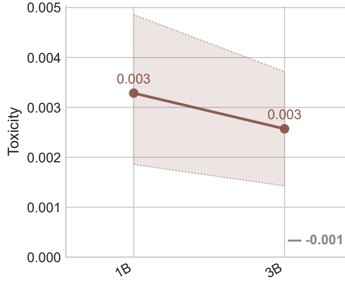
LLaMA-3.2
