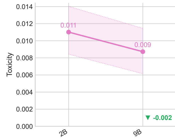
Gemma-2
