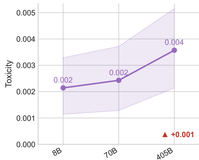
LLaMA-3.1
