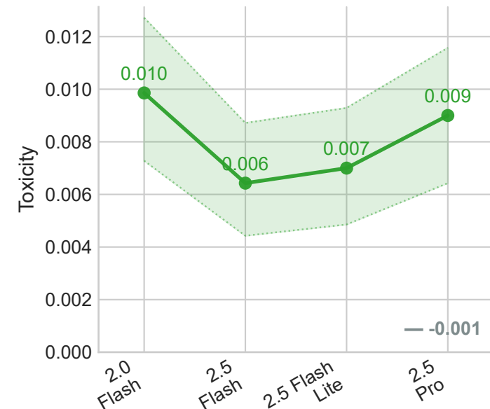
Gemini
