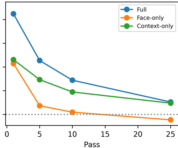
canonswap
