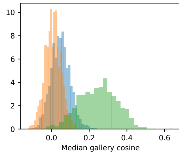
e4s
