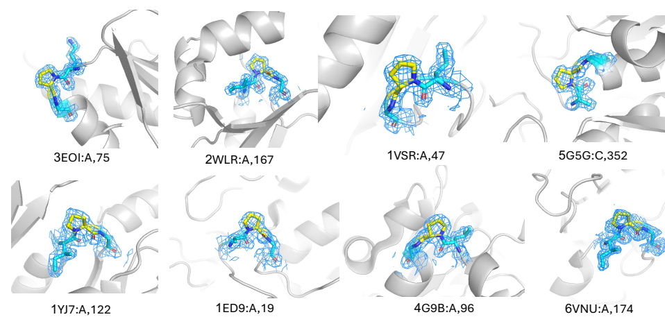
Turn P-CCC:P-CCG kde-l1(bw=10.0)
