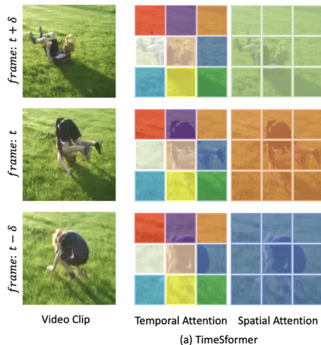
Figura 2.7: Ilustración de los mecanismos de atención de un TimeSformer
