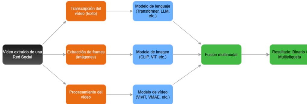
Figura 2.1: Flujo de procesamiento multimodal de vídeos (texto + imagen + vídeos)
