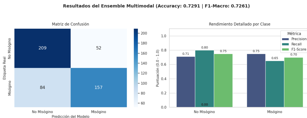
Figura 3.4: Resultados del Ensemble Multimodal contra el test estático
