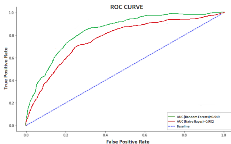
Figura 3.16: Curvas ROC de los modelos evaluados.
