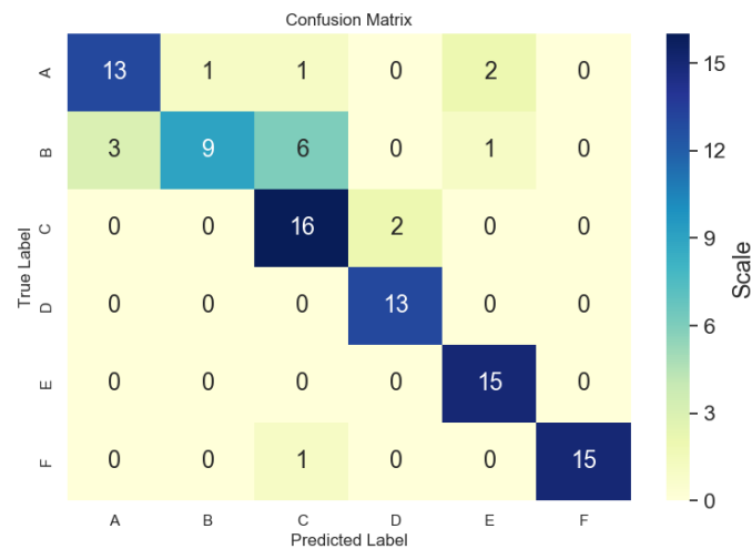
Figura 3.15: Matriz de confusión para el modelo RoBERTa.
