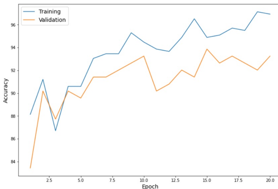
Figura 3.13: Evolución del entrenamiento monitorizada con TensorBoard.
