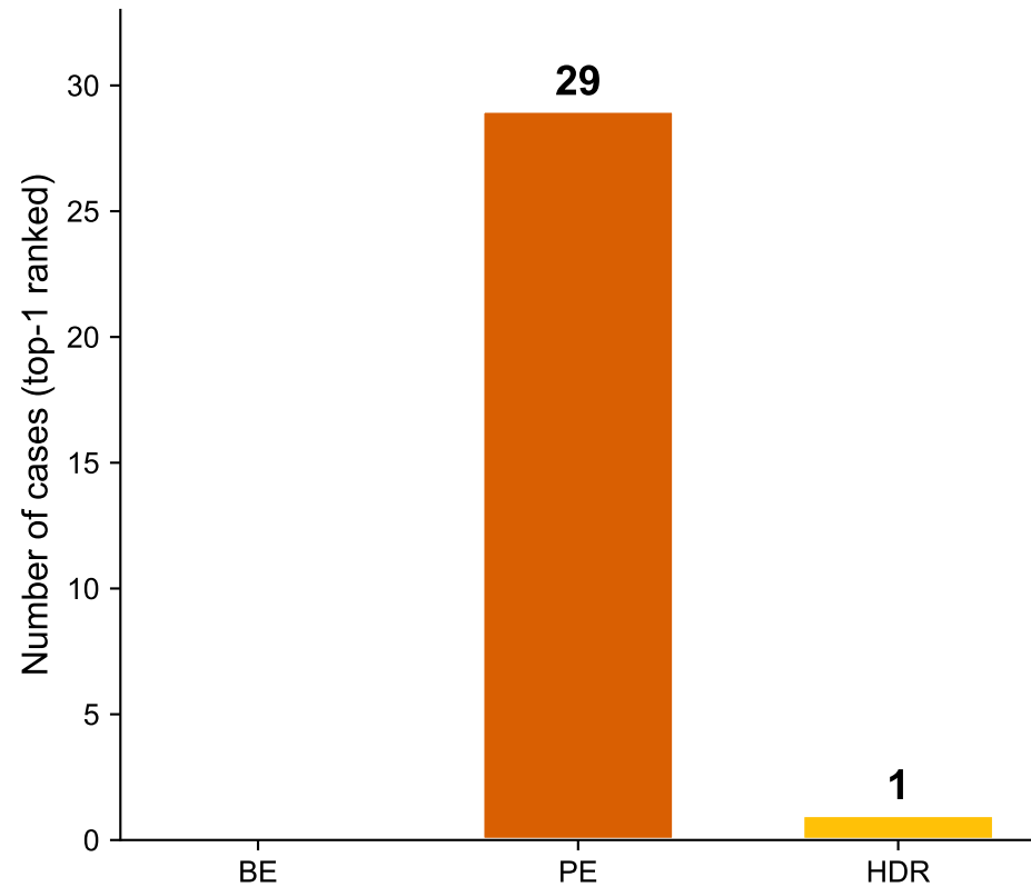
v2 (SpCas9 + ABE7.10)
