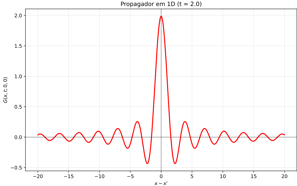
Figure 3: Função de Green (propagador) em 1D
