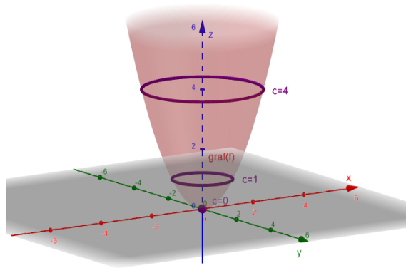
Figura 1.21: graf(f)
