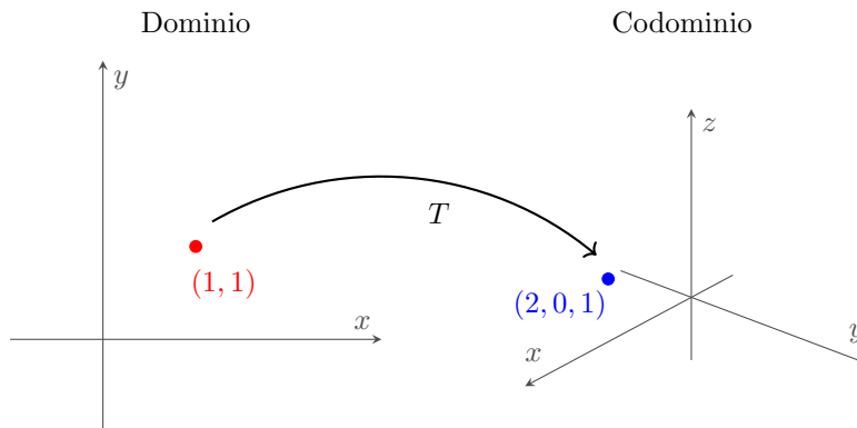
Figura 1.12: T como una relación entre \mathbb{R}^2 y \mathbb{R}^3 . Visualización de \mathbf{T}(1, 1) = (2, 0, 1)
