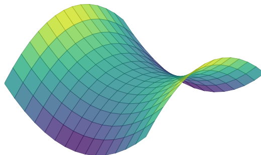
Superficie orientable
