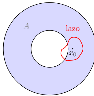
Conjunto NO simplemente conexo
