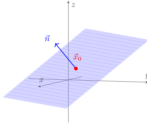
Figura 1.6: Ejemplo un plano \pi , con su punto de paso \mathbf{x}_0 y vector normal \mathbf{n} .
