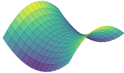
Superficie orientable
