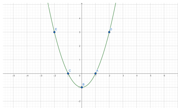
Figura 1.17: Grafica de f(x) .
