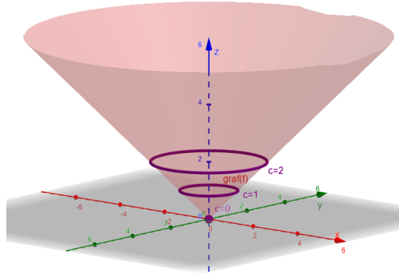
Figura 1.22: Conjuntos de nivel y graf(f)
