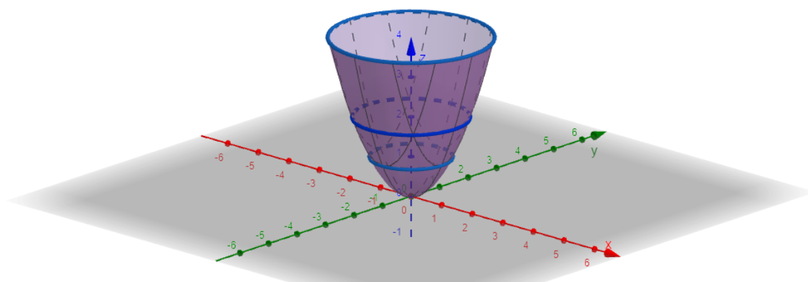
Figura 1.18: Gráfica de h y conjuntos de nivel tomando c=\{1,2,4\}
