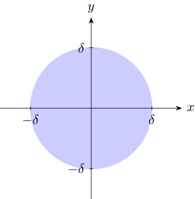
Bola con norma 2
