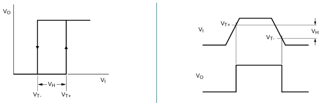
Slika 3.4. Prijenosna karakteristika (lijevo) i primjer rada sklopa (desno) [3]
