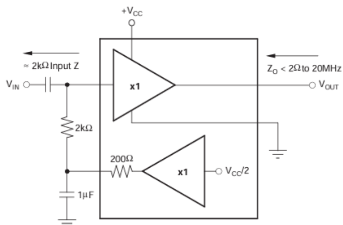
Slika 3.2. Blok shema naponskog sljedila BUF602ID [6]
