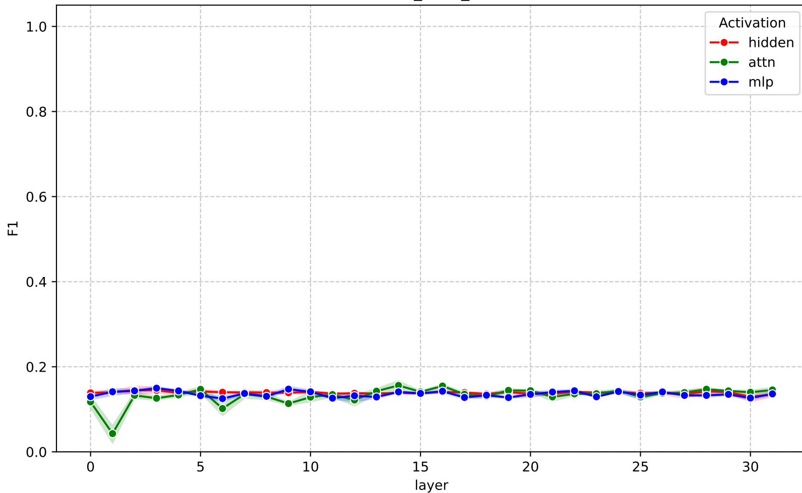
F1 across layers - gemma-3-4b-it (cross_cquad_ffn)
