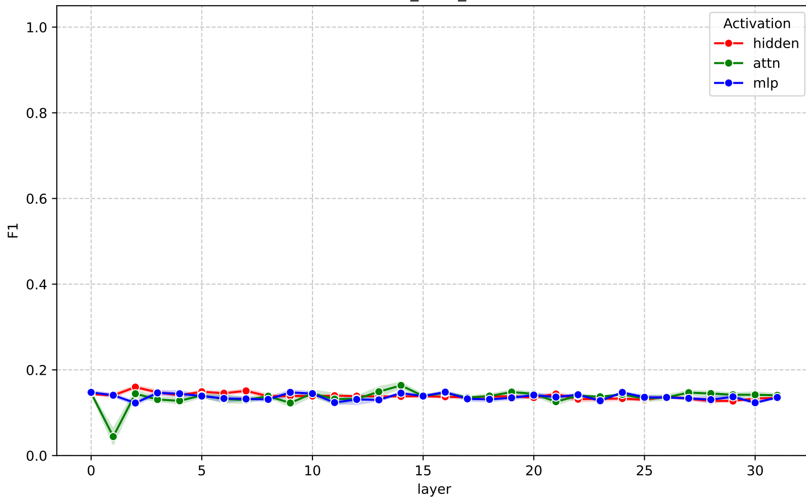
F1 across layers - gemma-3-4b-it (cross_cquad_svm)
